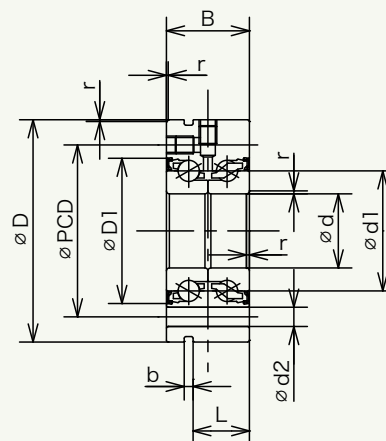
A-O-A'截面
